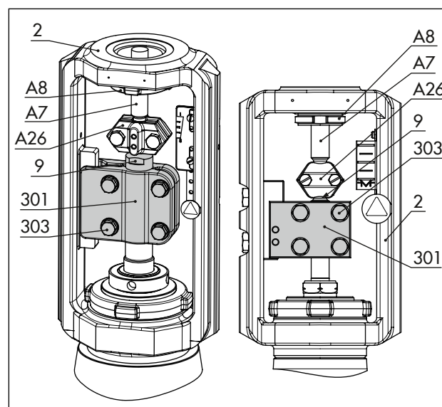
Fig. 9 : Dispositif de blocage : exécution standard (à gauche), exécution spéciale (à droite)
