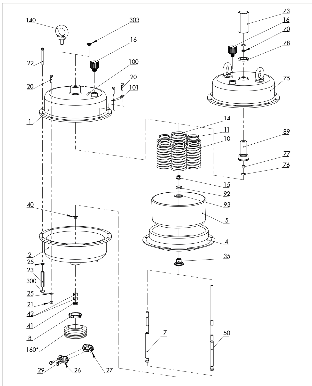
Fig. 17 : Servomoteur type 3271, 1000 cm 2
