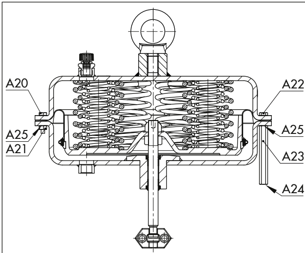
Fig. 10 : Servomoteur avec vis et écrous de serrage (exemple illustré)
