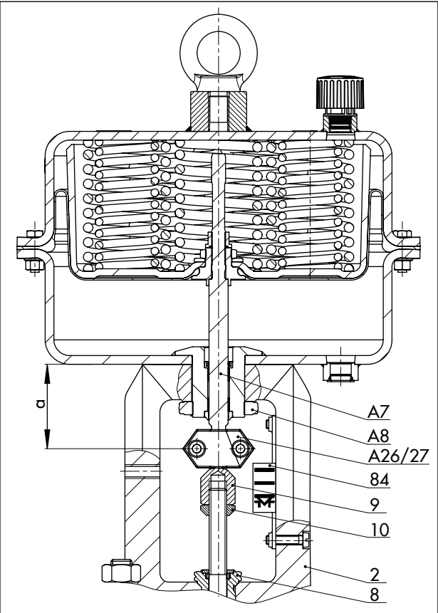
Fig. 8 : Servomoteur pneumatique type 3271 monté sur une vanne linéaire
