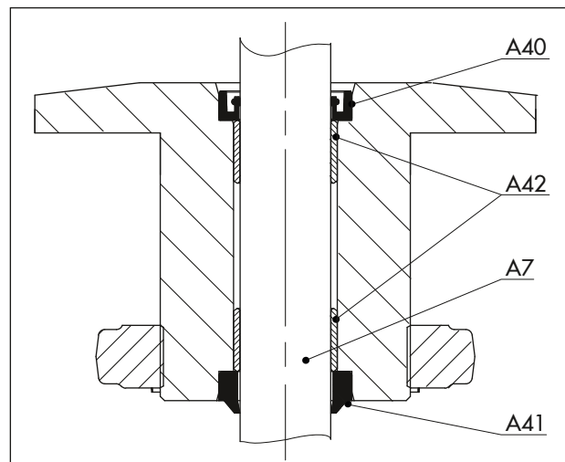
Fig. 15 : Type 3271 Étanchéité de la tige de servomoteur
