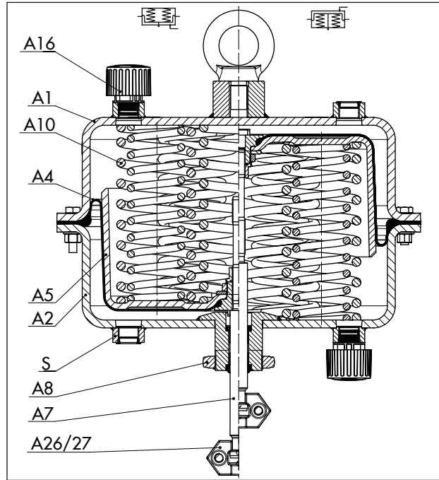
Fig. 2 : Servomoteur pneumatique type 3271, exemple illustré avec surface de 1000 \text{ cm}^2
