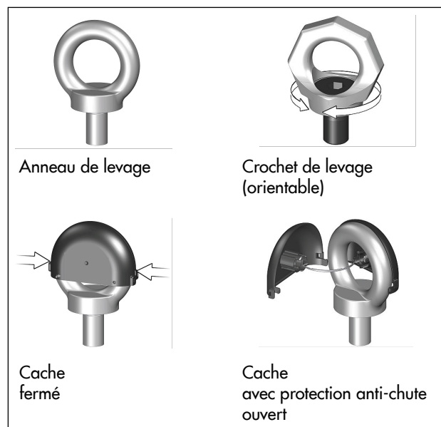
Fig. 5 : Protection anti-chute au niveau de l'anneau de levage/crochet de levage
