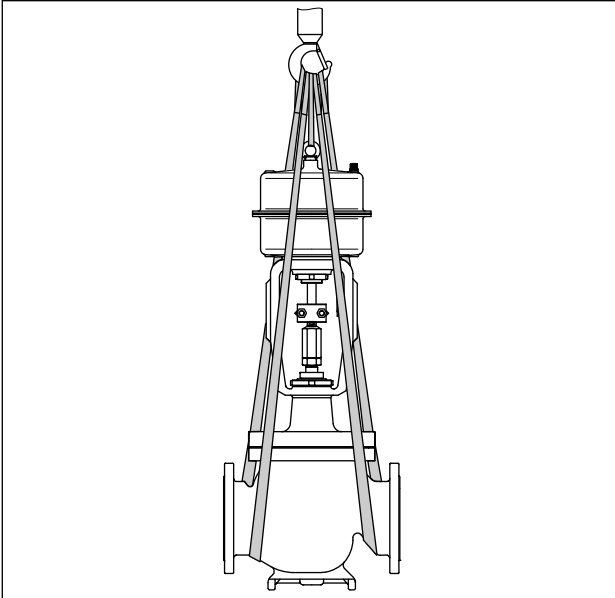
Fig. 7 : Points de levage sur la vanne de régulation (exemple)
