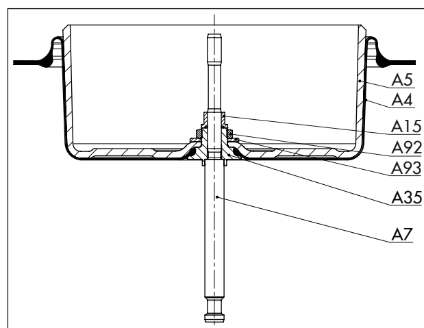
Fig. 12 : Ordre des pièces dans le sens d'action TS (1000 cm²)
