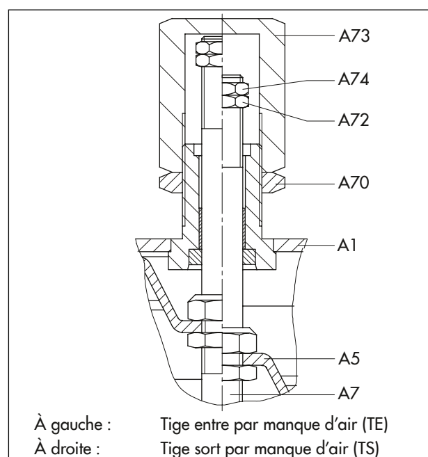
Fig. 11 : Limitation de course
