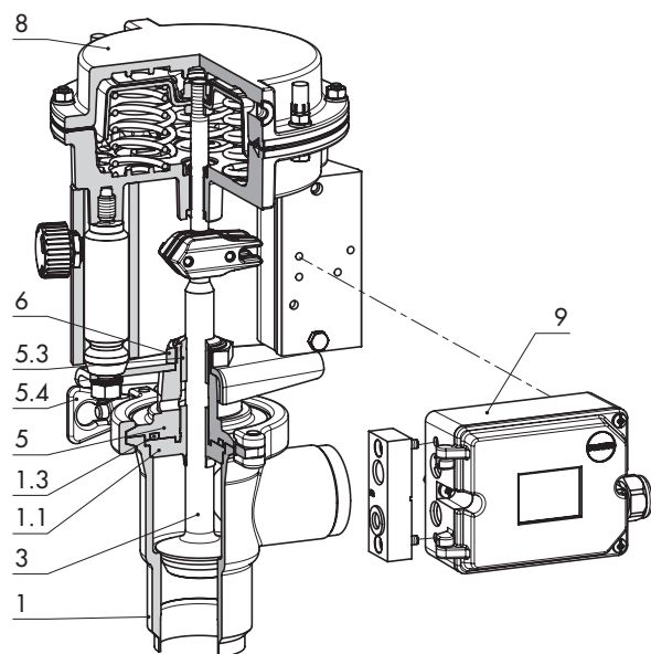
Fig. 3 : Vanne de régulation type 3347 avec servomoteur pneumatique type 3372 d'une surface de 120 cm 2 et positionneur type 3725
