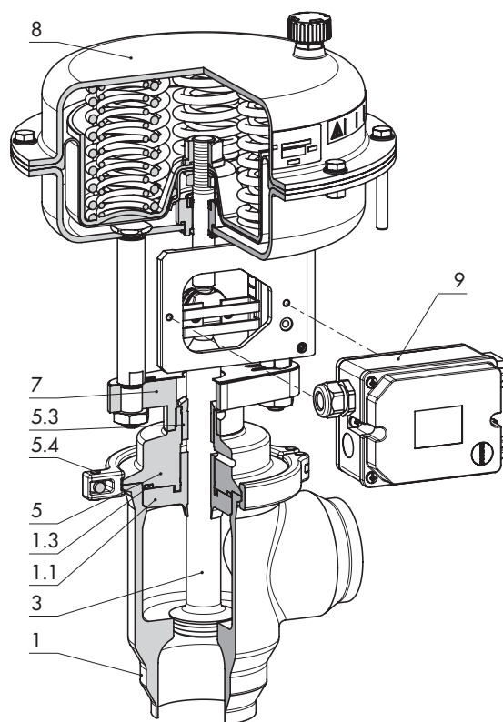
Fig. 4 : Vanne de régulation type 3347 avec servomoteur pneumatique type 3372 d'une surface de 350 cm 2 et positionneur type 3725
