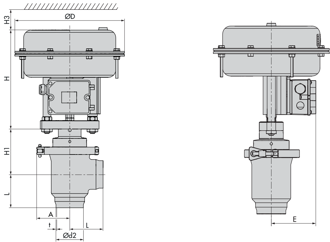
Vanne à passage équerre type 3347 avec servomoteur pneumatique type 3372, 350 cm 2 et positionneur type 3725
